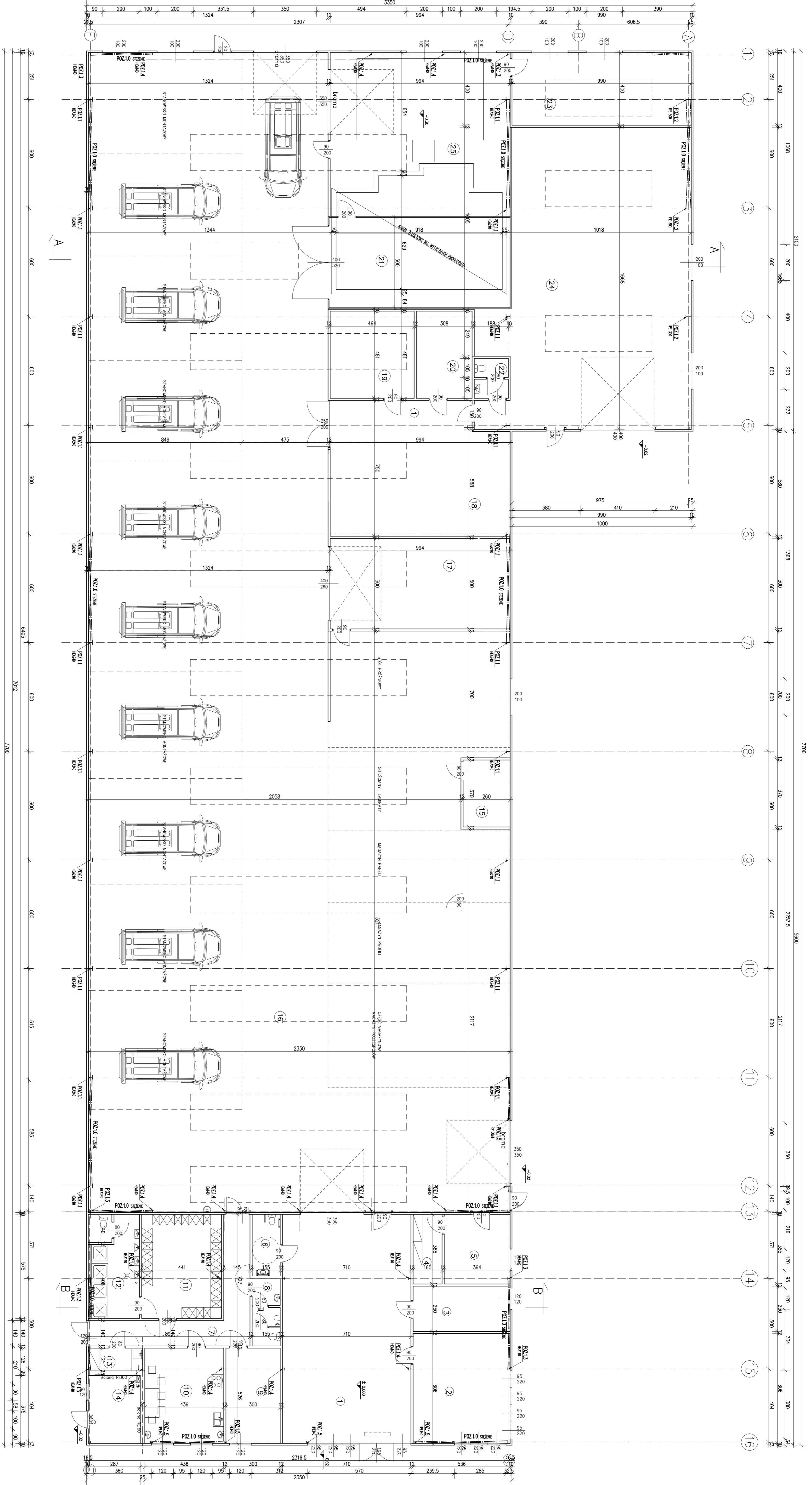
RZUT PARTERU 1:100
